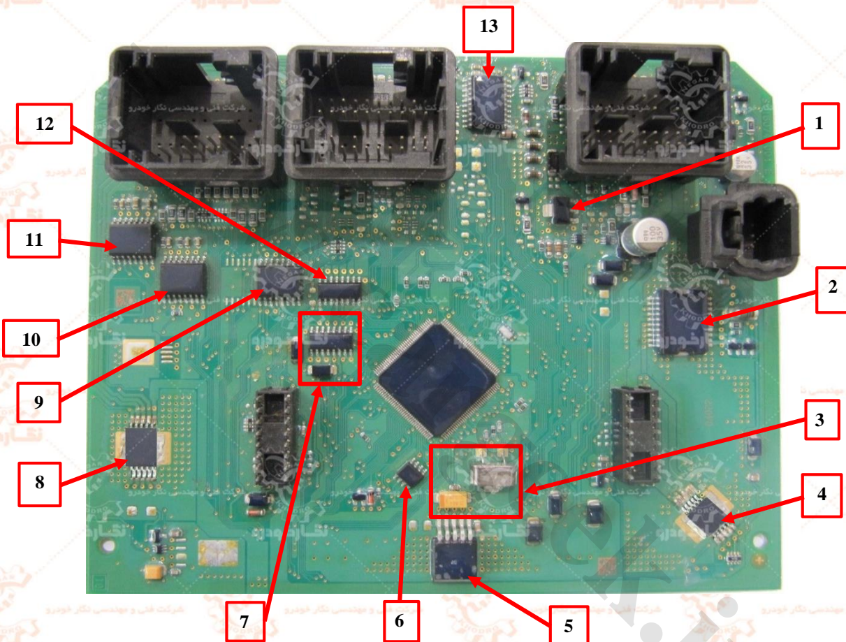
نمای کلی جلو بخش A نود BSI
